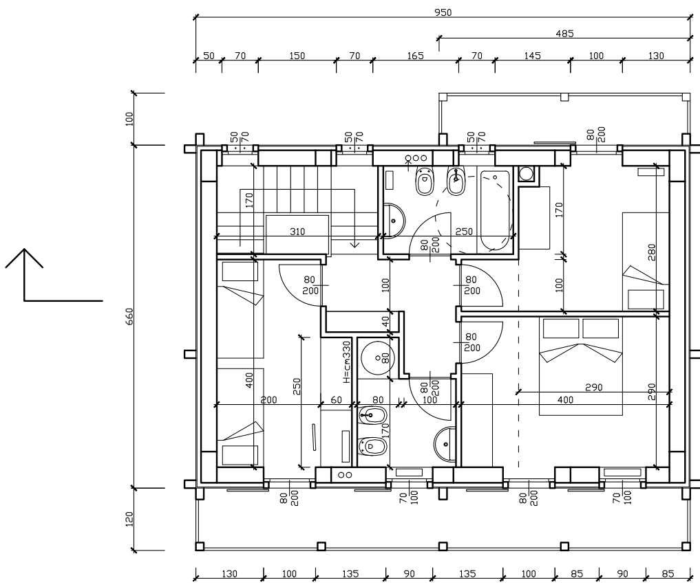
Piano primo
