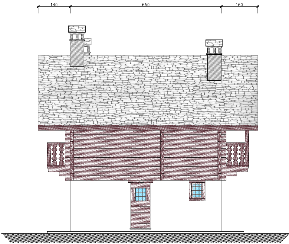
Prospetto Nord
