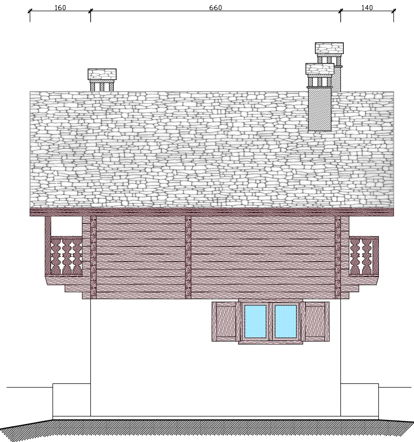
Prospetto Sud
