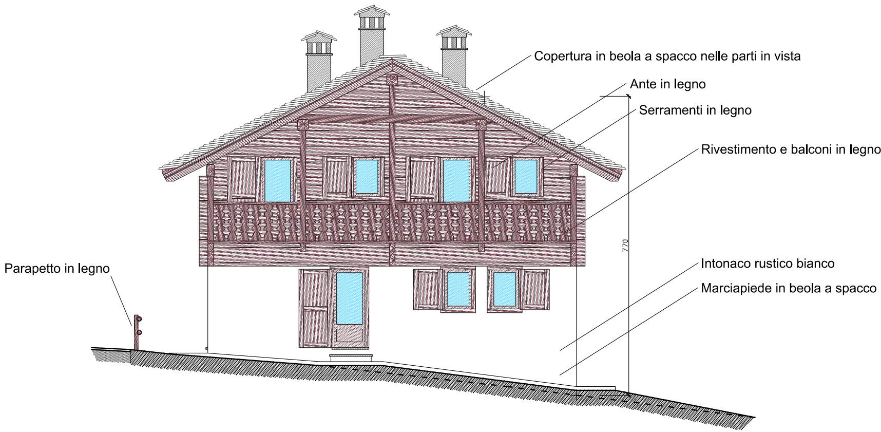
Prospetto Ovest
