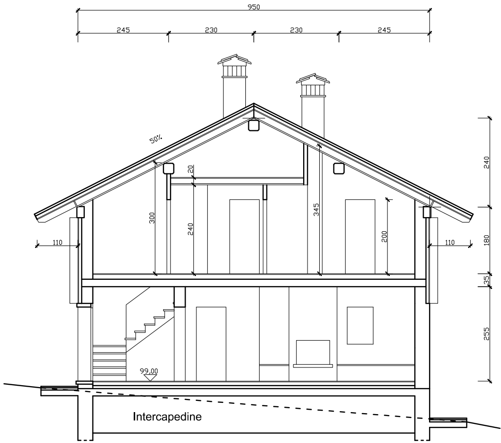
Sezione
