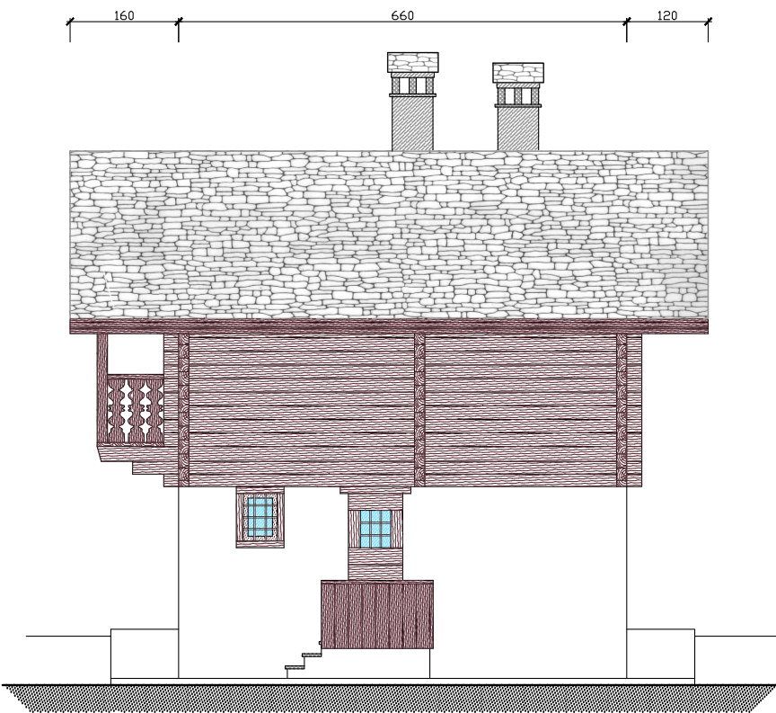
Prospetto Sud
