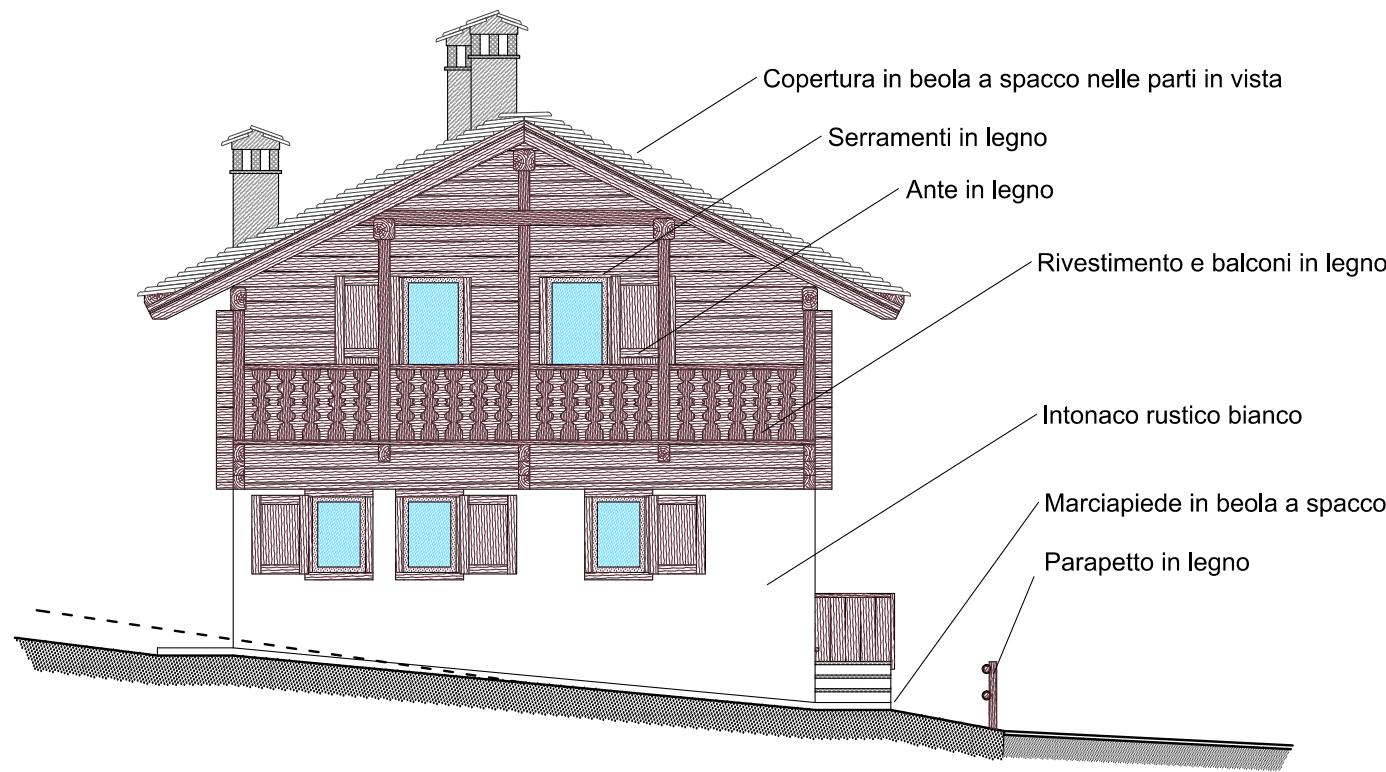
Prospetto Ovest
