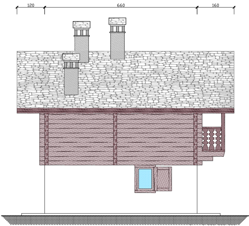
Prospetto Nord
