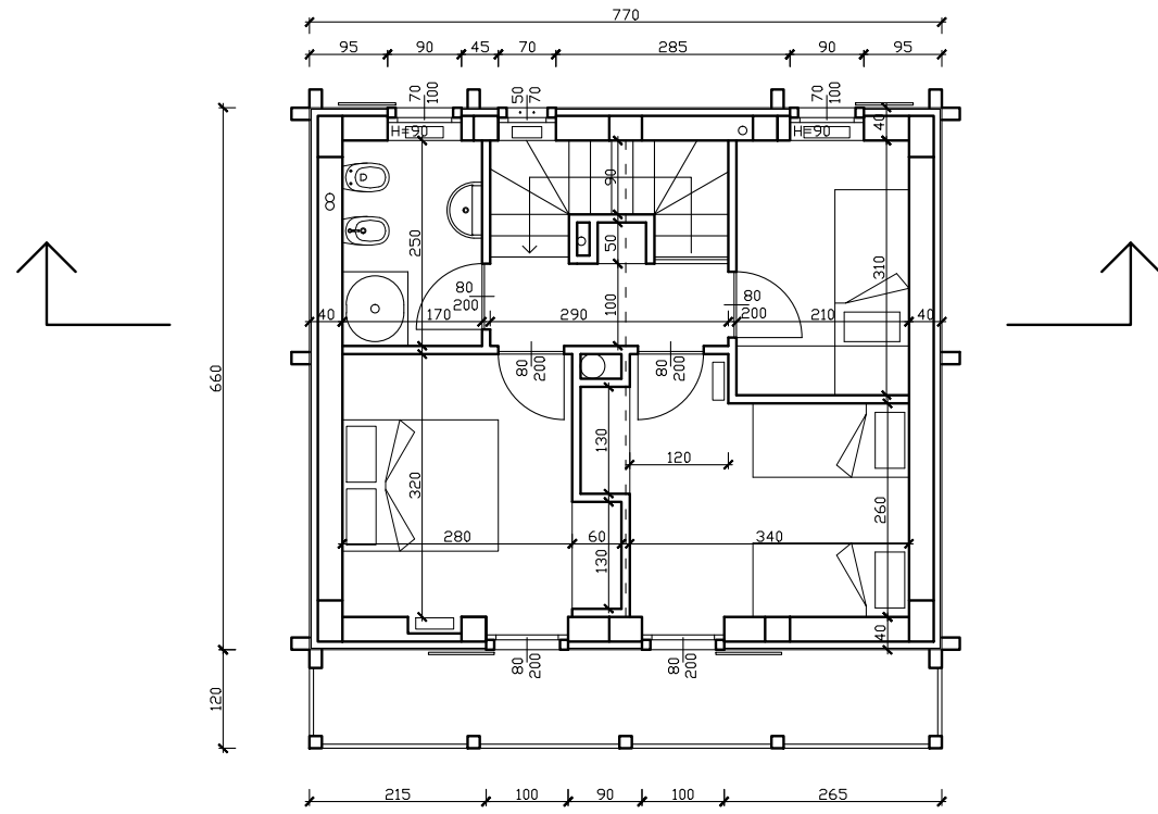
Piano primo
