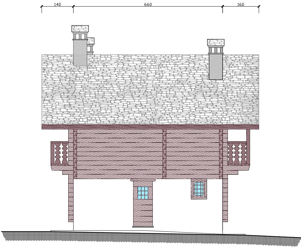
Prospetto Nord
