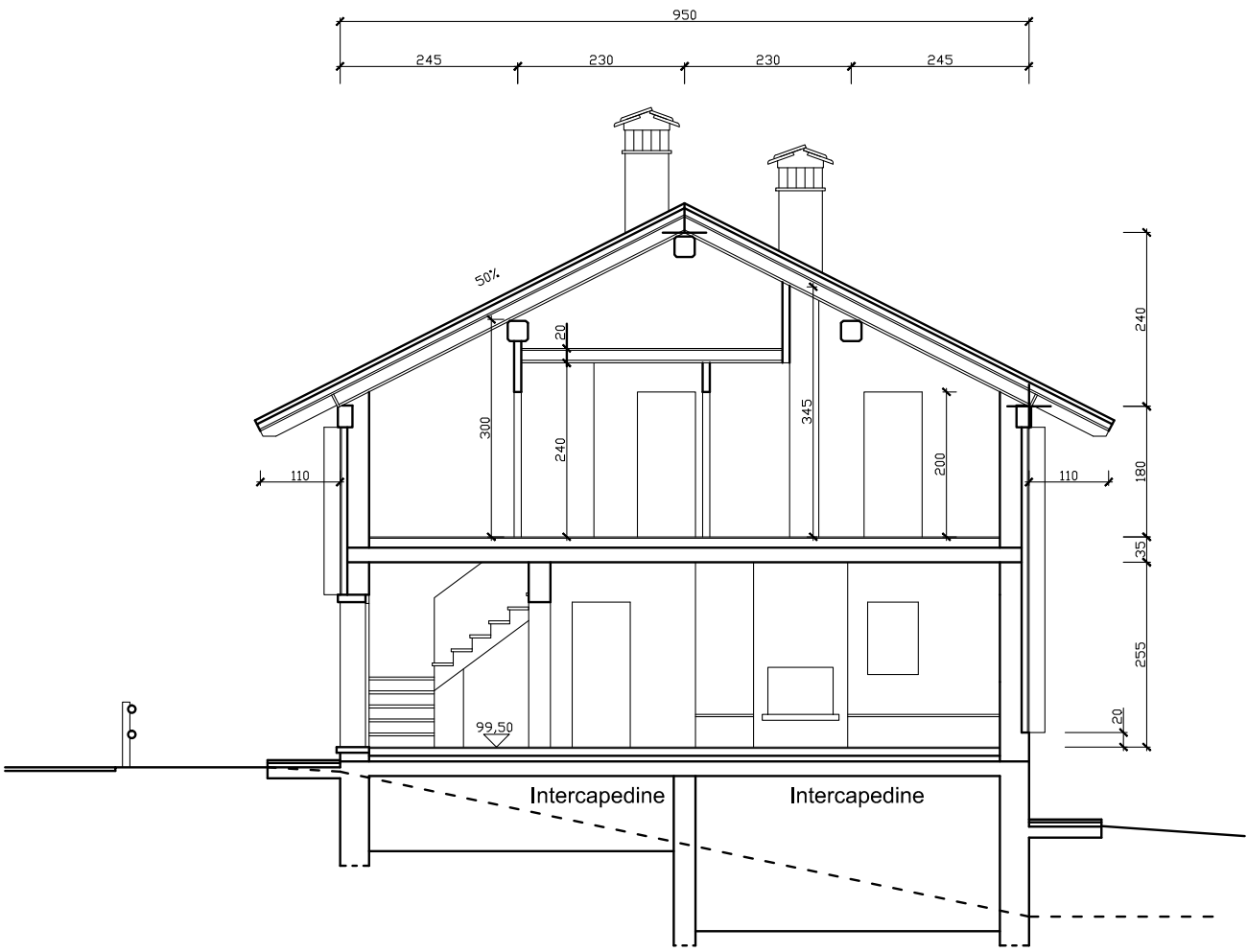
Sezione
