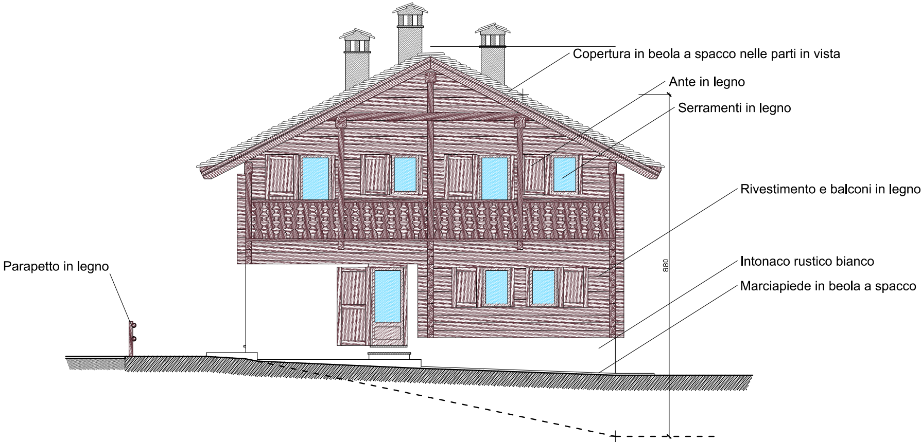
Prospetto Ovest
