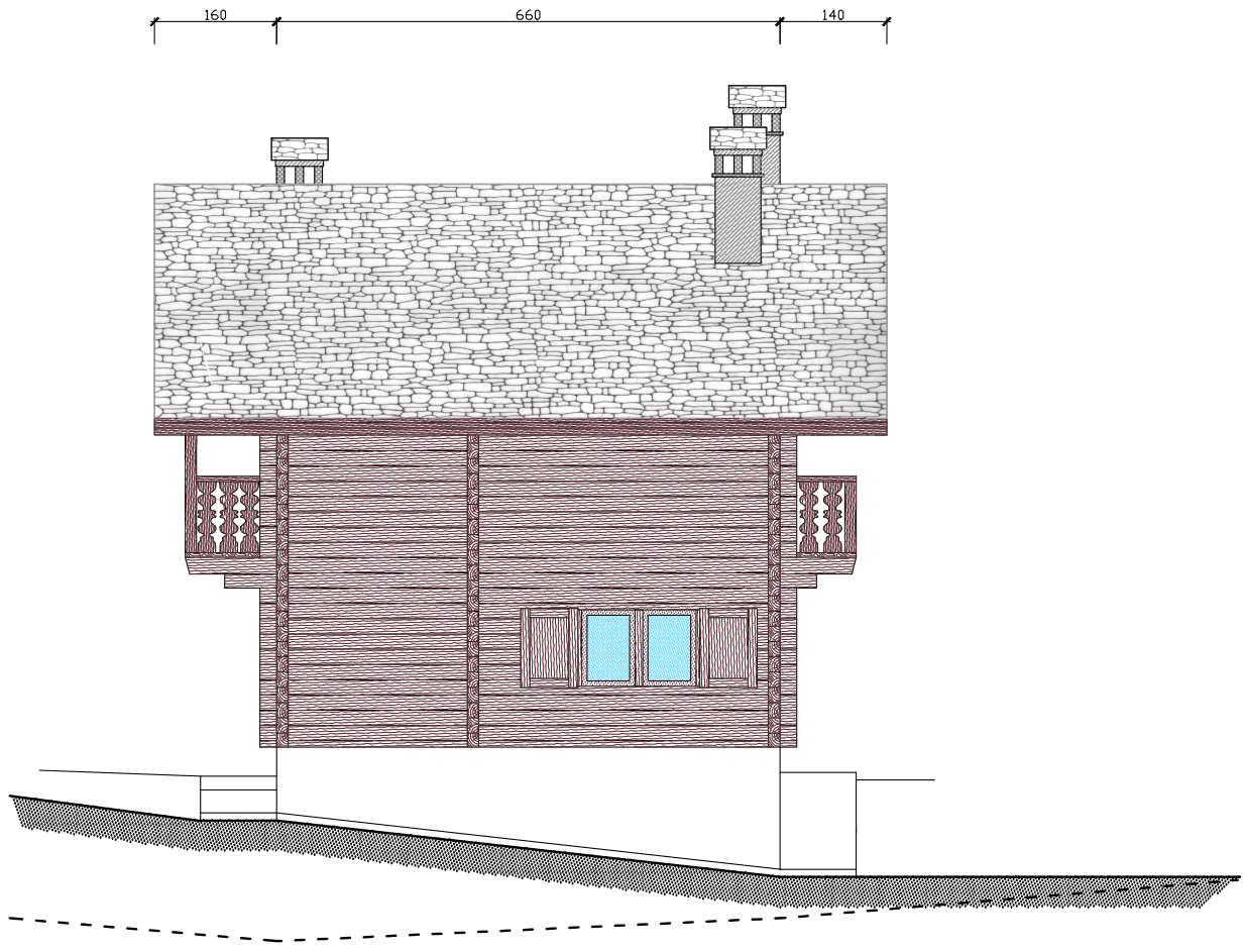
Prospetto Sud
