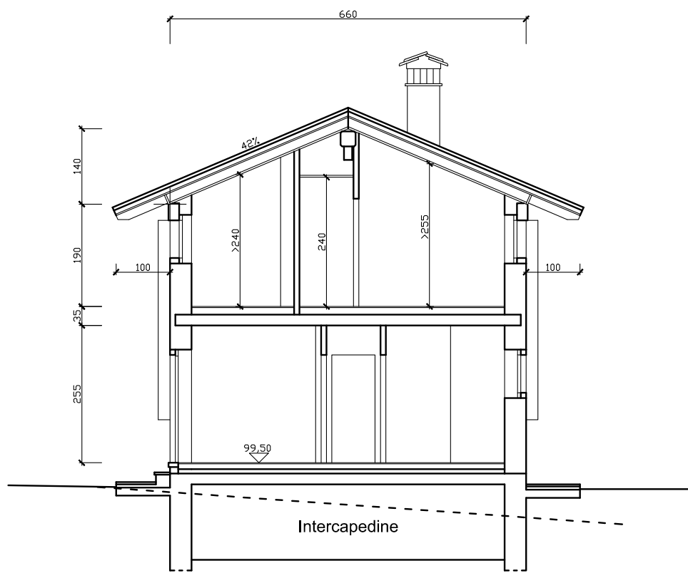
Sezione
