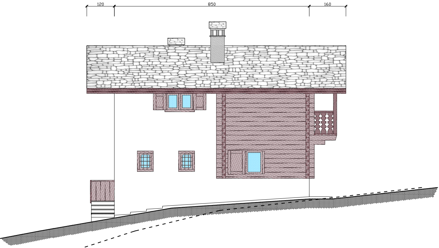
Prospetto Nord
