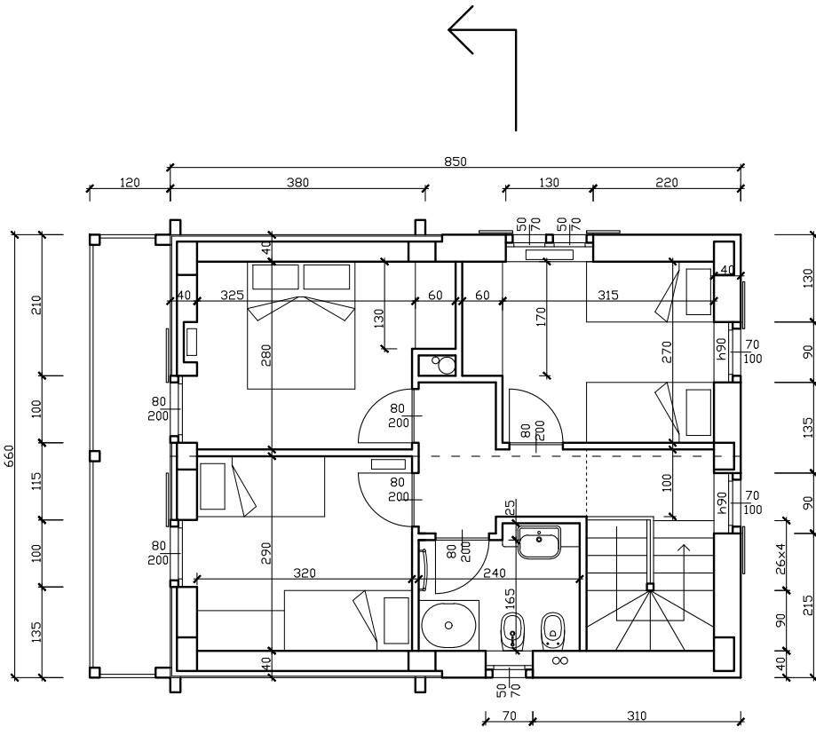
Piano primo
