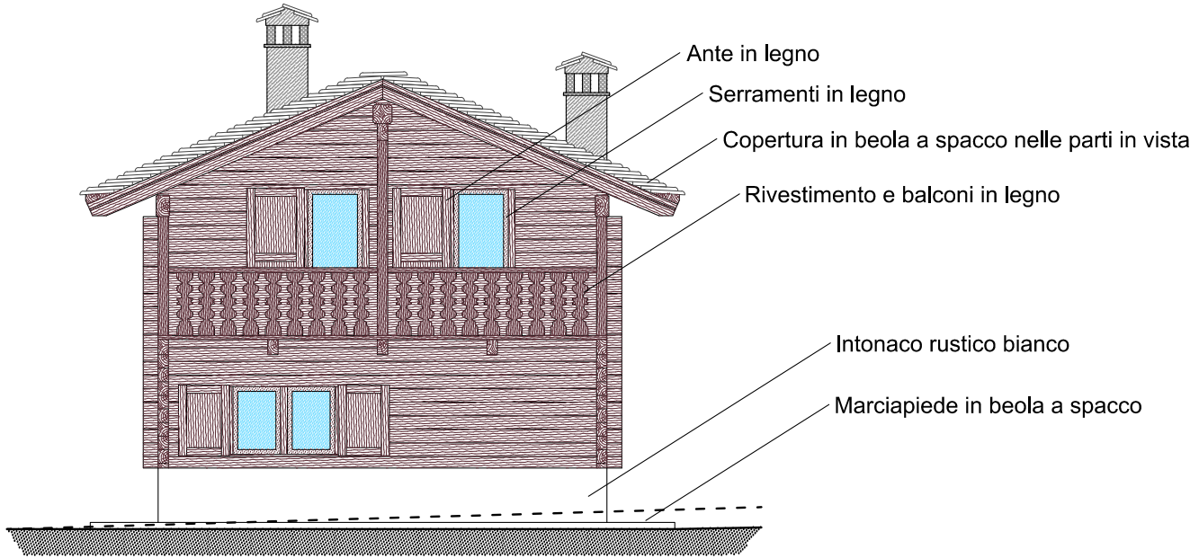
Prospetto Ovest
