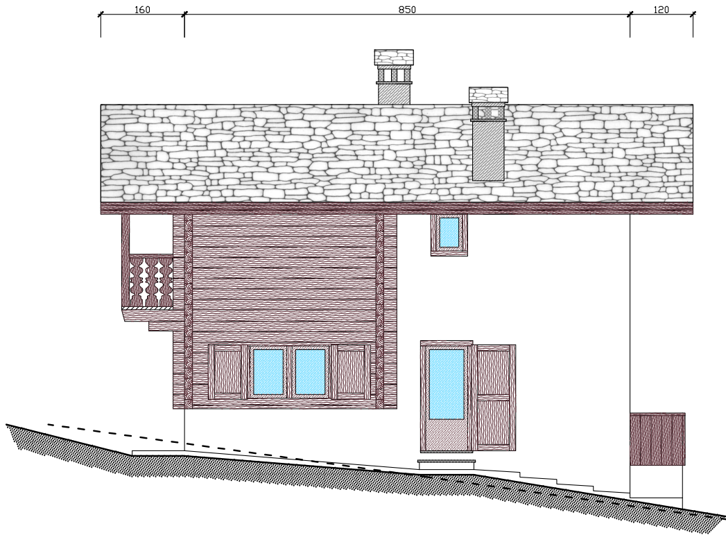
Prospetto Sud
