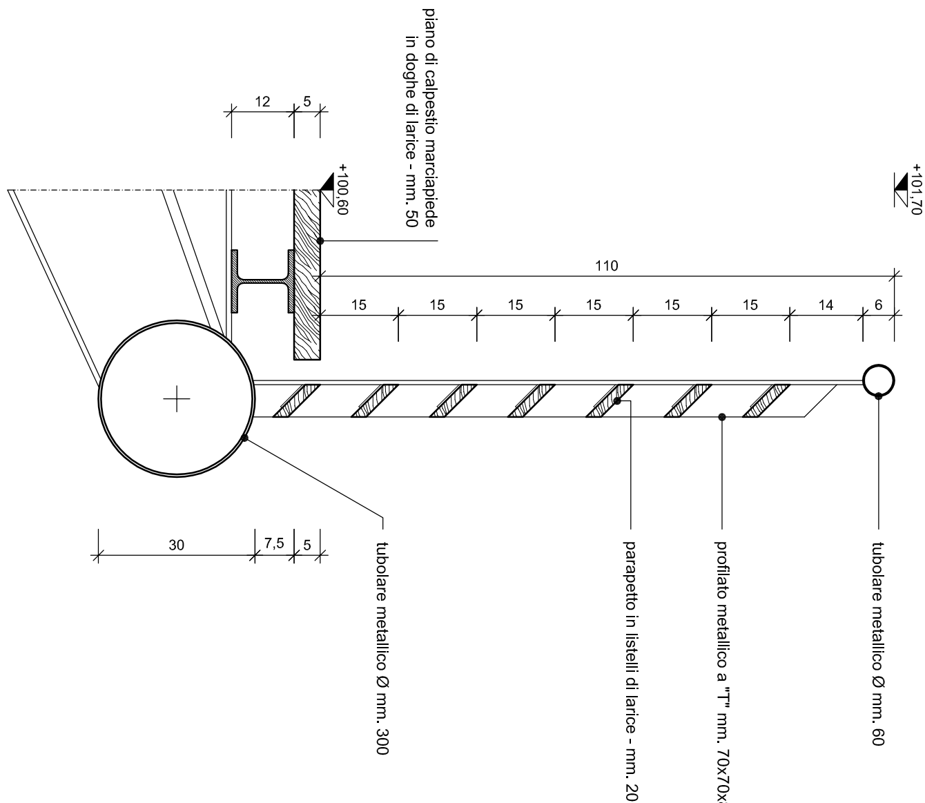
PARTICOLARE PARAPETTO - scala 1:10
